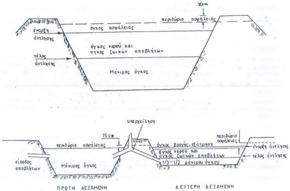
Σχήμα 7. Απεικόνιση επιμέρους όγκου υγρών που περιέχονται σε μονή και διπλή AXAD (πηγή: Εργαστήριο Γεωργικών Κατασκευών του ΓΠΑ).
